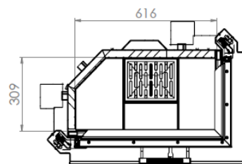
PRZĘKRÓJ A-A
